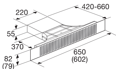
Vue latérale plan de travail 600 mm Combinaison HR0003 et HR0011
