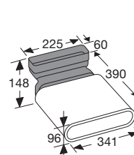
Zijaanzicht met liggend plasmafilter en adapter
