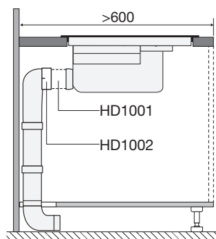
Zijaanzicht verdiept werkblad
